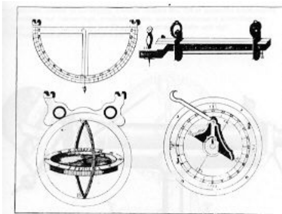
Winkelmessinstrumente der Markscheider. Aus: M. Magold, Lehrbuch der Polygonometrie und Markscheiderkunst, 1804
