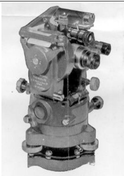
Teodolit med optiskt lod från Hilgur&Watts
